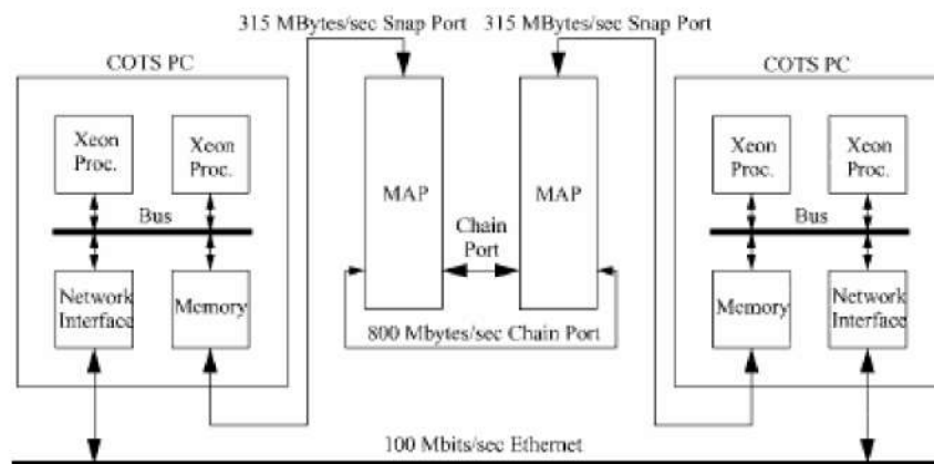
شکل ۳- معماری SRC-6e
